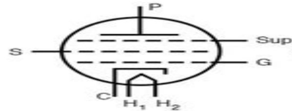
Pentode
