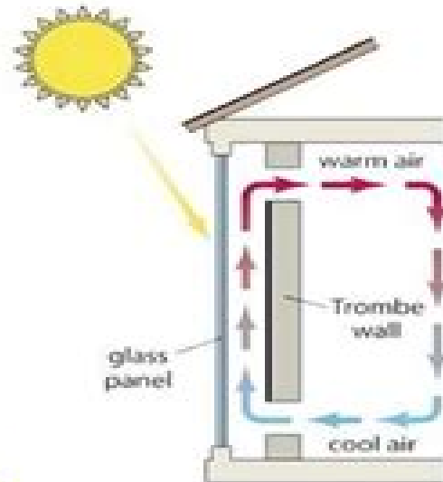
Trombe wall
