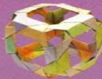
FORMAS GEOMÉTRICAS
