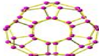
42 ( D_5 )
