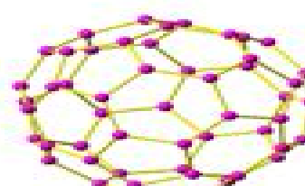
52 ( T )
