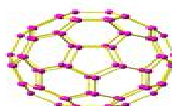
60 ( I_h )
