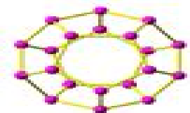
20 ( I_h )
