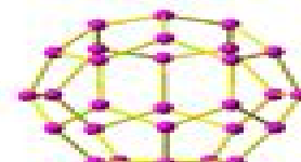
28 ( T_d )
