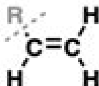
alkene (-alkenyl)
