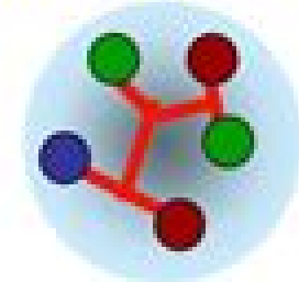
Pentaquark
