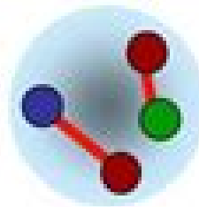
Tetraquark
