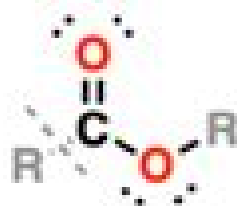
ester
