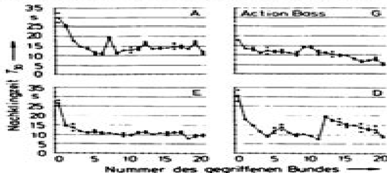
Fig. 1. Nachklingen T_{30} für 30 dB Pegelabfall.
