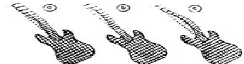
Fig. 2. Ausgewählte Schwingungsformen, der unverformte Baß ist gestrichelt.
