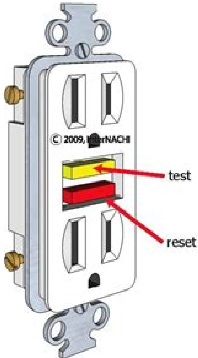
RECEPTACLE
