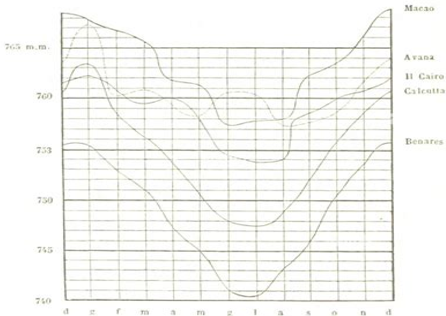
Fig. 29. — Variazioni mensili del Barometro nelle regioni calde.
