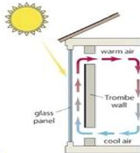
Trombe wall
