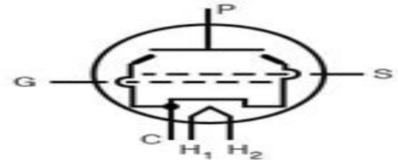
Thyratron
