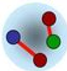
Tetraquark
