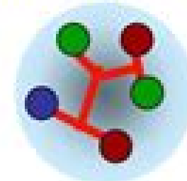
Pentaquark
