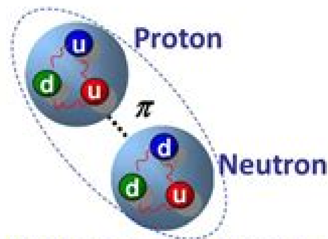
Deuteron: p-n molecule
