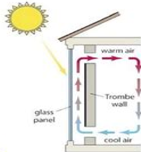
Trombe wall
